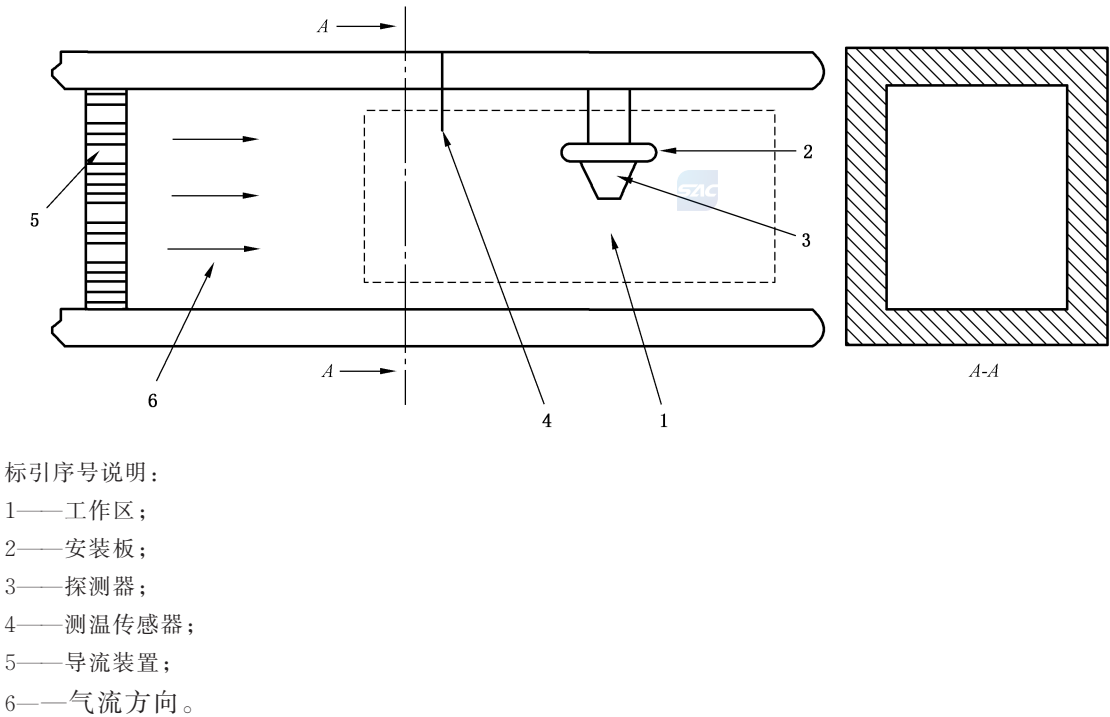
图 A.1 标准温箱工作区域示意图
